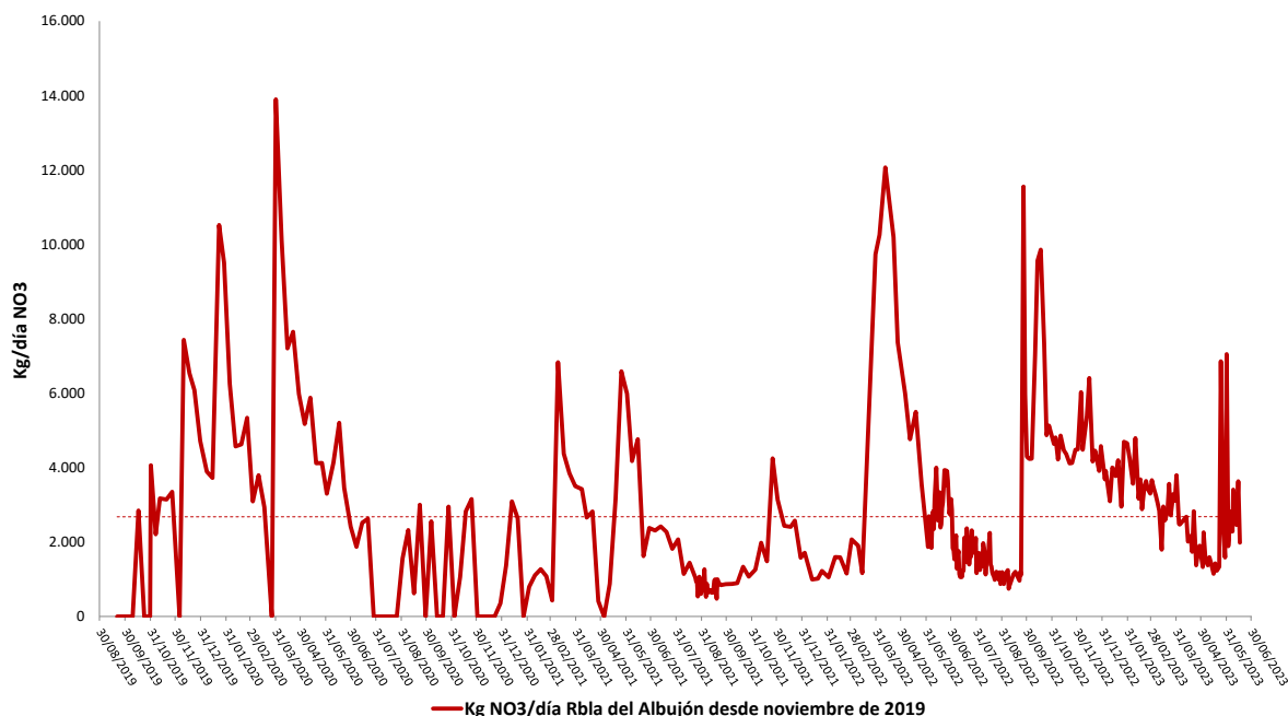
Evolución de los promedios de nitratos (Kg/día) desaguado en la desembocadura del Albuñón
