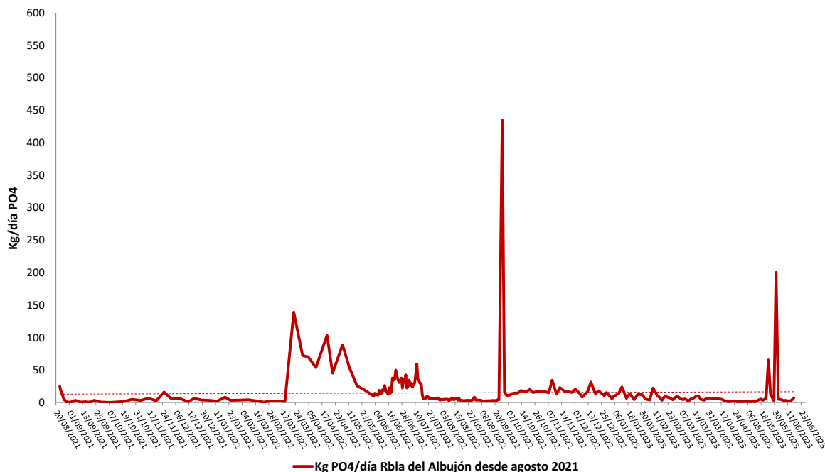
Kg PO 4 /día DESAGUADO POR LA DESEMBOCADURA DE LA RBLA. DEL ALBUJÓN DESDE AGOSTO 2021
