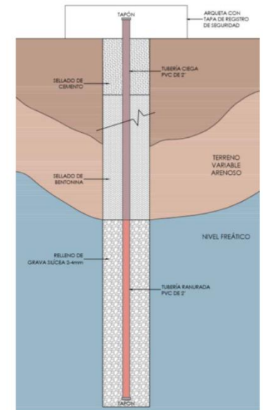
Sección tipo de sondeo
